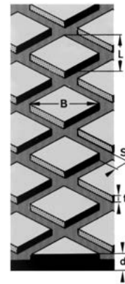
UNIGRIP 60
