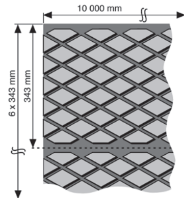
REMAGRIP 70 – SL
