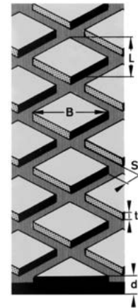
REAGRIP 60 HR
