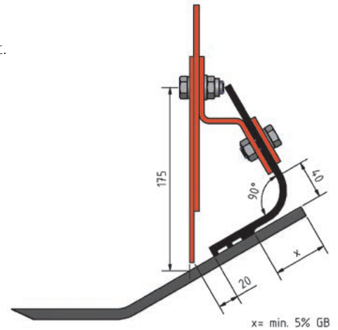
REMASKIRT CB 195
